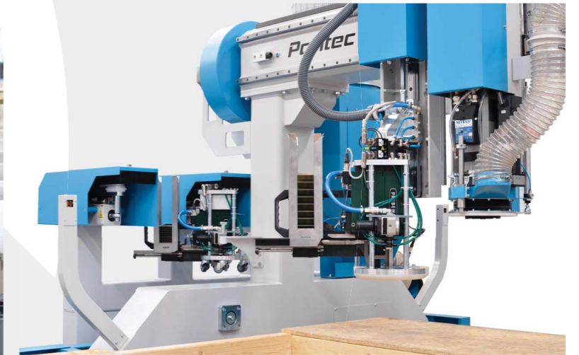
Automatisches Linearmagazin für pneumatische Werkzeuge
