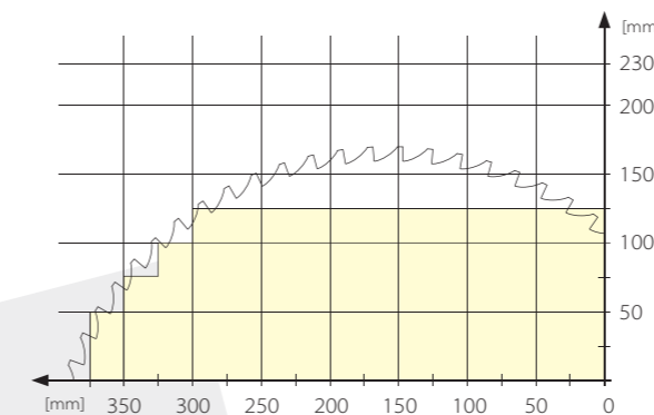
Schnittschema für Crossline 500
