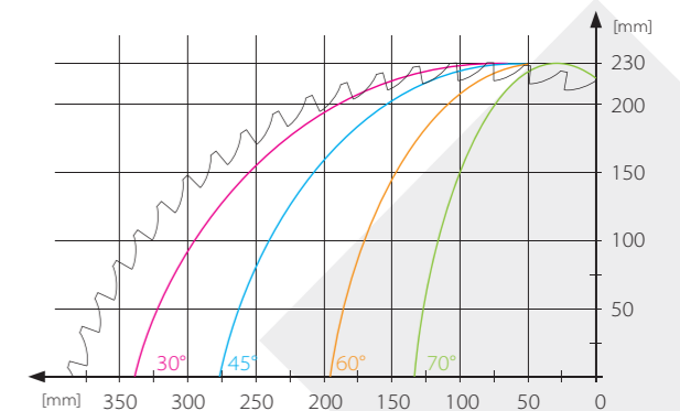
Schnittschema für Crossline 650
