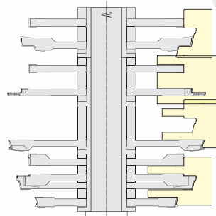
Nástroje pro TEMAC E s programovatelnými pozicemi a rozděleným opracováváním
