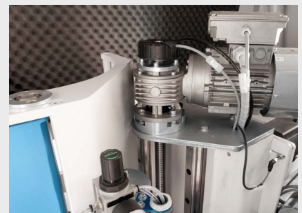
Elektronické nastavování – verze E Electronic positioning – E series
